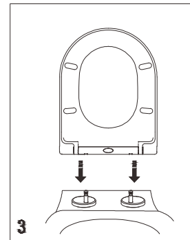
3 Klik de zitting op de bevestigingspinnen
